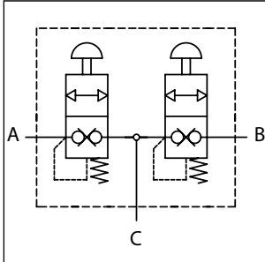
BLOCCO 57 (Manifold 57)
